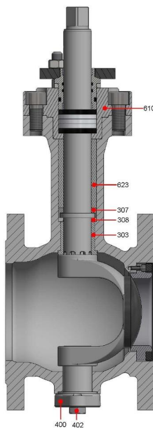
Bild 4: 82.7-01, DN 150, TA-Luft
