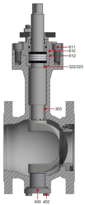
Bild 5: 82.7-02, DN 150, TA-Luft
