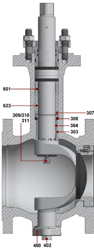
Bild 3: 82.7, DN 150, TA-Luft
