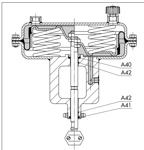
図 28: アクチュエータ軸シール（タイプ 3277）
