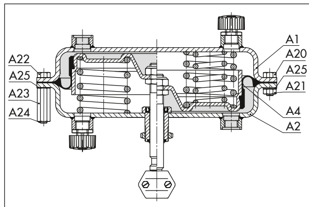
図 18: クランピングナットとボルト付きアクチュエータ
