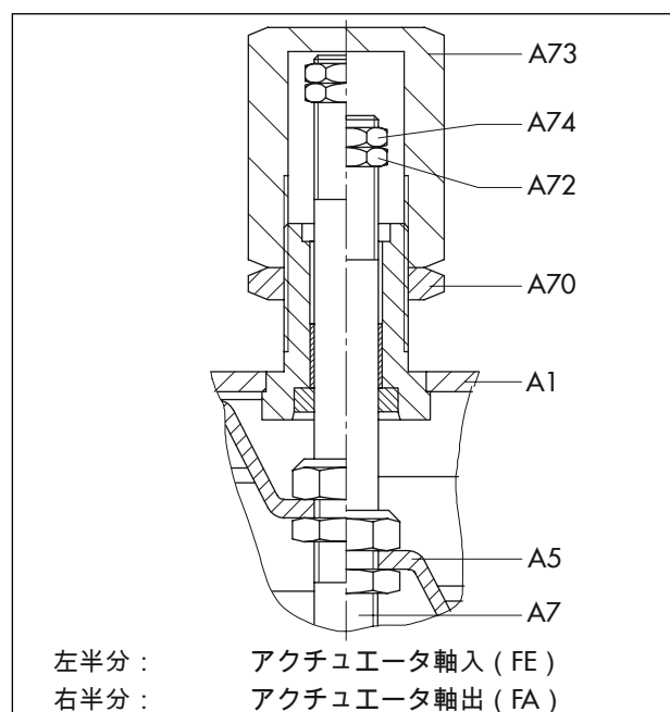
図 19: トラベルストップ
