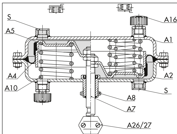
図 2: アクチュエータ タイプ 3271（操作部面積 350 cm 2 の例）
