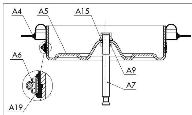
図 23: 「軸出」作動方向の場合の部品配列 (240、350、700 cm 2 )
