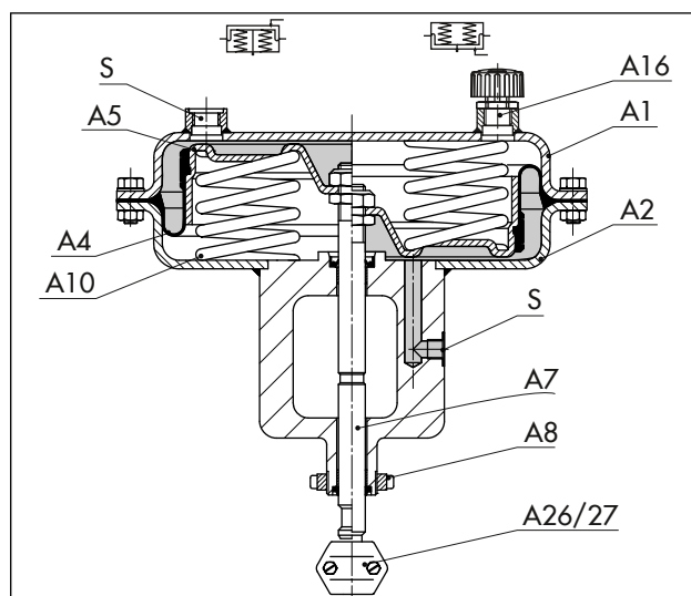
図 22: アクチュエータ タイプ 3277 (操作部面積 350 cm 2 の例)
