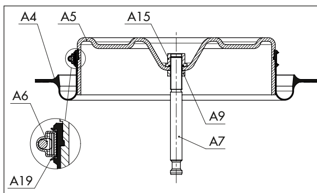
図 25: 「軸入」作動方向の場合の部品配列 (240、350、700 cm 2 )
