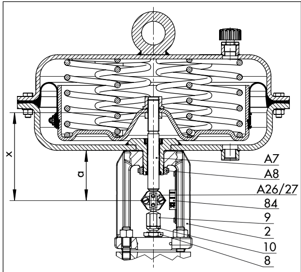
図 16: グローブ弁に取り付ける空気式アクチュエータ タイプ 3271
