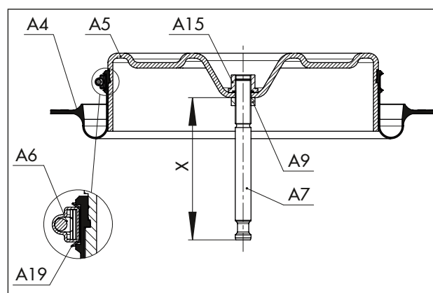
図 29: 作動方向が「軸入」の場合の部品配列
