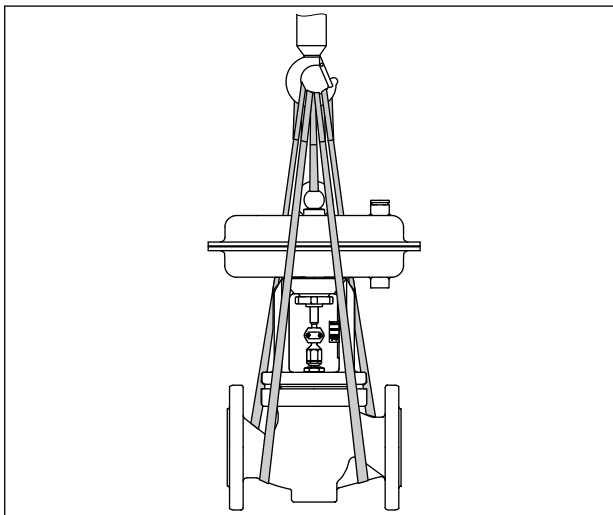
図 15: 調節弁の吊上げポイント（図は例）
