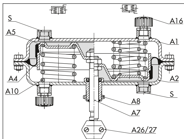
図 21: アクチュエータ タイプ 3271 (操作部面積 350 cm 2 の例)
