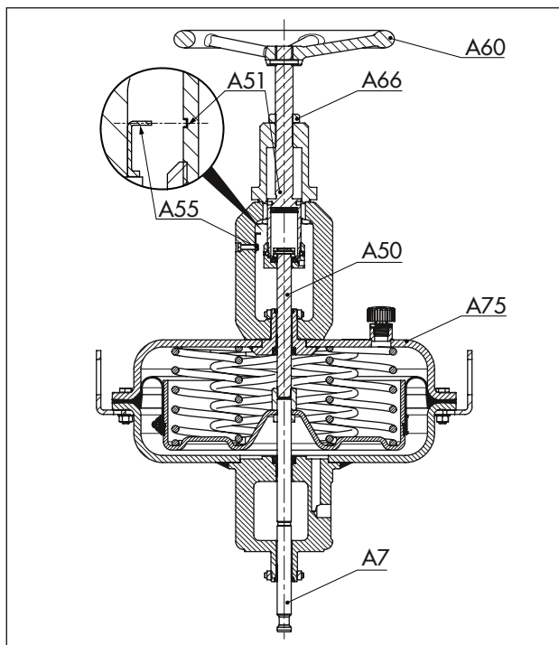
図 20: 空気式アクチュエータ タイプ 3277、手動ハンドル付き
