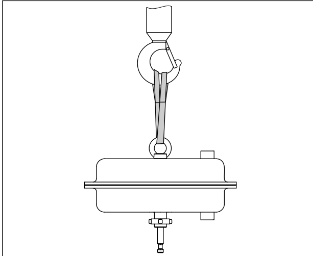
図 14: アクチュエータの吊上げポイント
