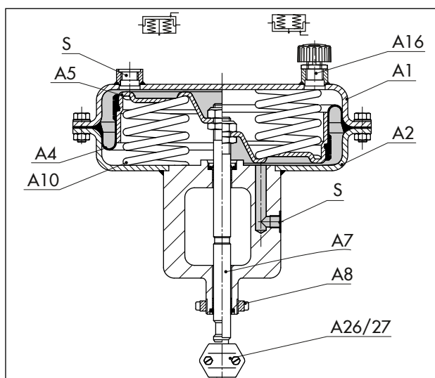
図 3: アクチュエータ タイプ 3277（操作部面積 350 cm 2 の例）
