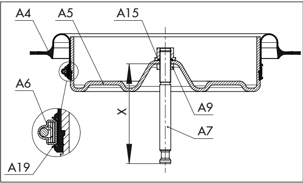
図 30: 作動方向が「軸出」の場合の部品配列
