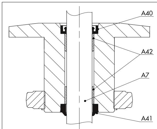
図 27: アクチュエータ軸シール（タイプ 3271）
