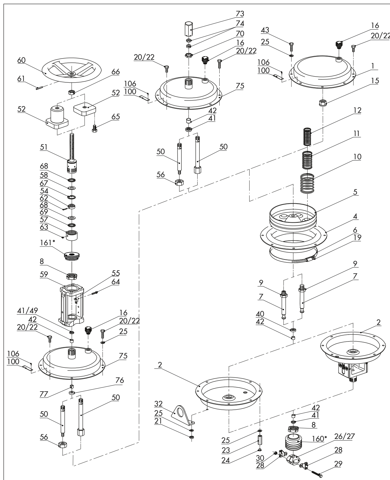
図 32: アクチュエータ タイプ 3271/3277 (240/350/700 cm²)
