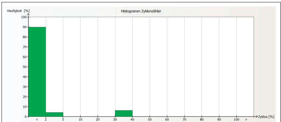
Bild 5: Diagnose > Beobachterfunktionen > Histogramm Zyklenzähler
