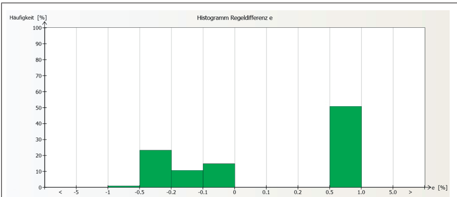
Bild 4: Diagnose > Beobachterfunktionen > Histogramm Regeldifferenz e
